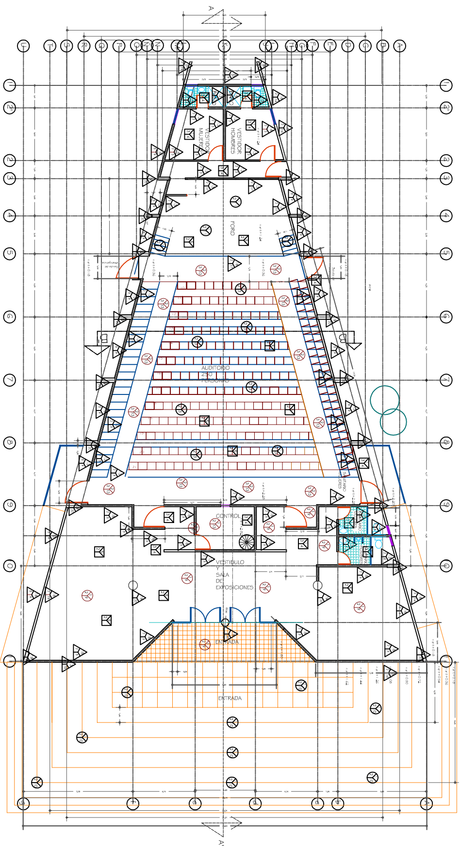
PLANTA ARQUITECTONICA
