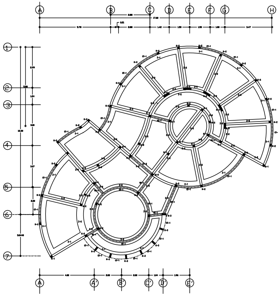
PLANTA DE CIMENTACION ESCALA 1 : 5 0
