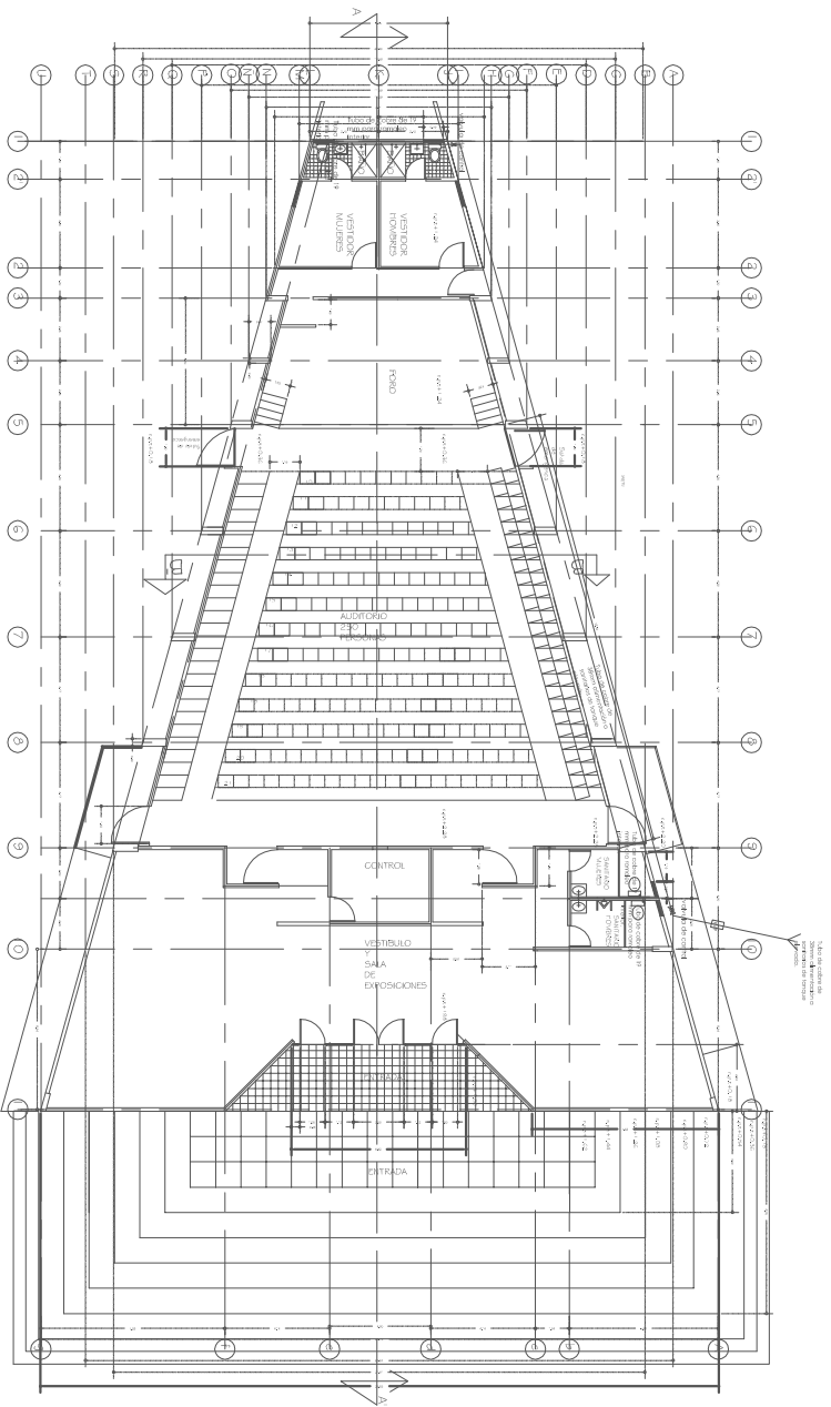
PLANTA ARQUITECTONICA
